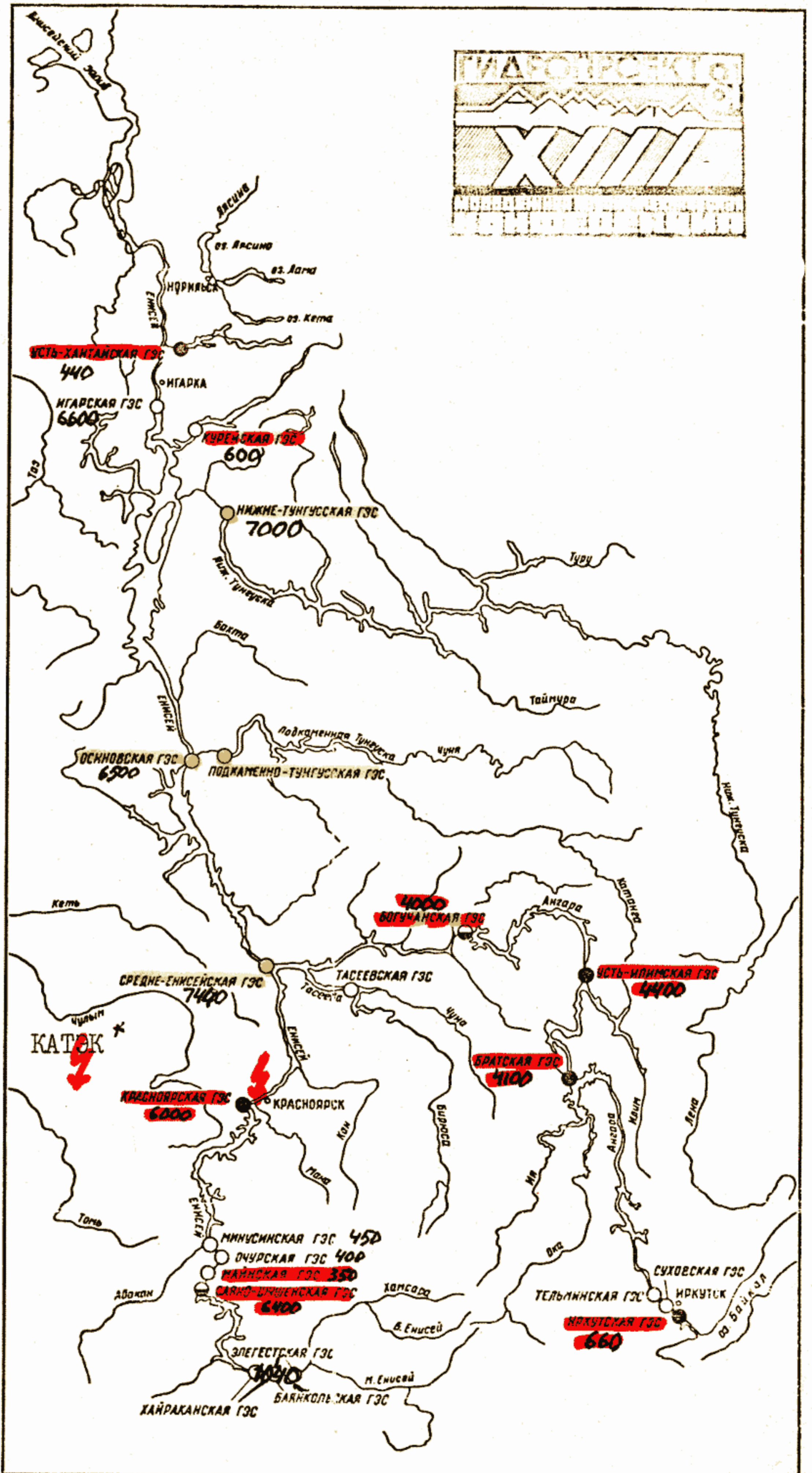
Схема размещения ГЭС на Енисее и его притоках
